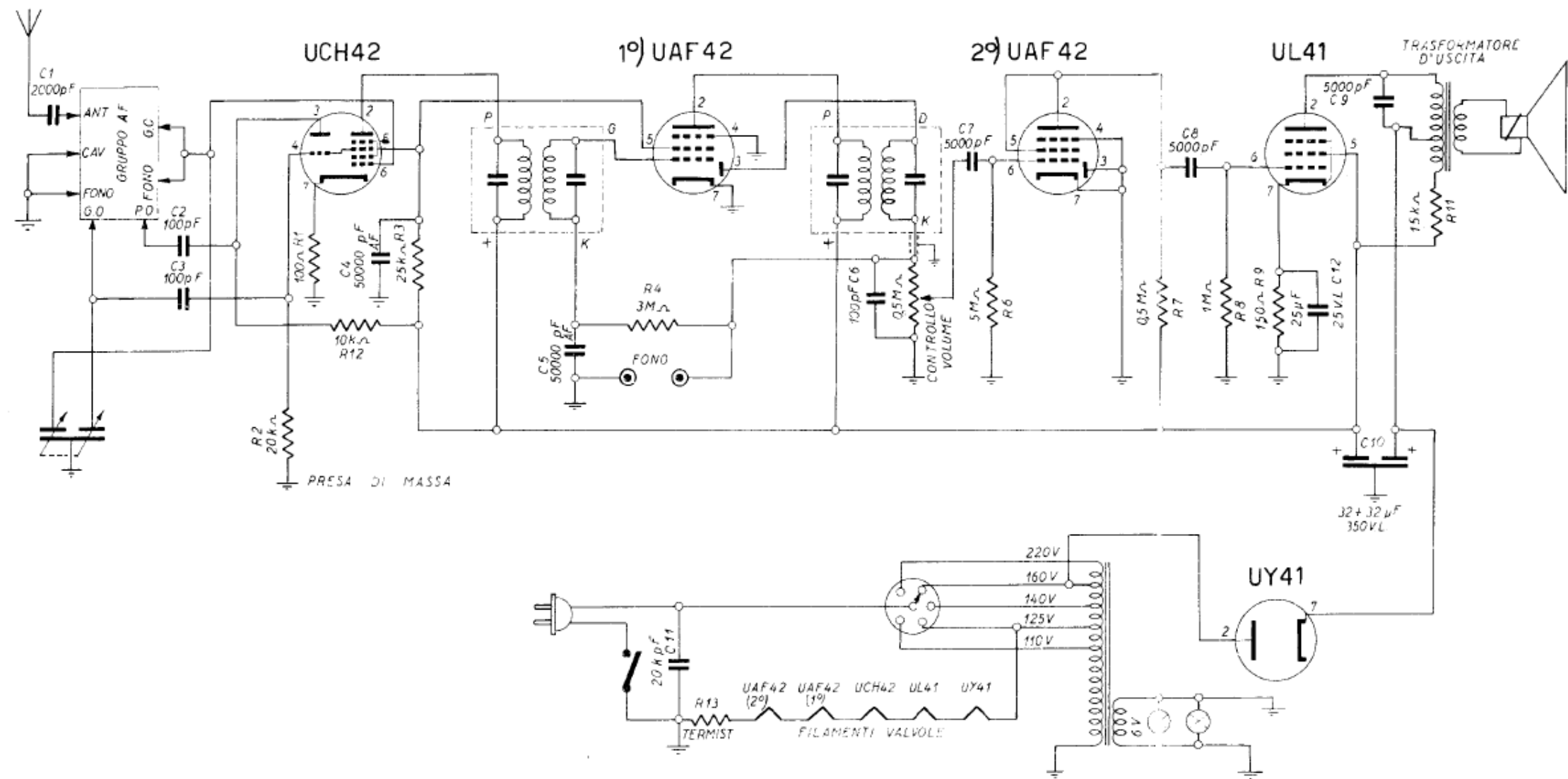
— Schema dell'apparecchio « Cosetta ».
